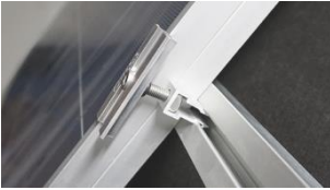
D. Skjut intill mittklämma mot solcellspanel.
