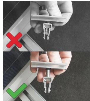
Insexskruv på mittklämma får EJ vara för långt gängad genom clips.
