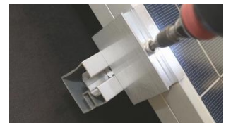
F. Skjut intill ändklämma mot solcellspanel och drag åt. Åtdragningsmoment 12 Nm
