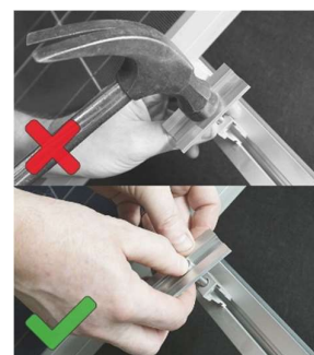
Använd EJ våld för att montera mittklämma.
