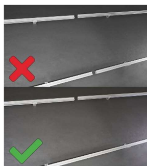
Skarvar på skenor skall förskjutas och får EJ placeras under samma solcellspanel.
