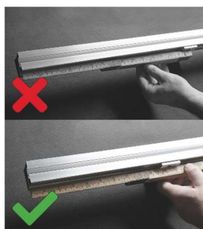
Överhäng på skena får EJ vara mer än 250 mm.
